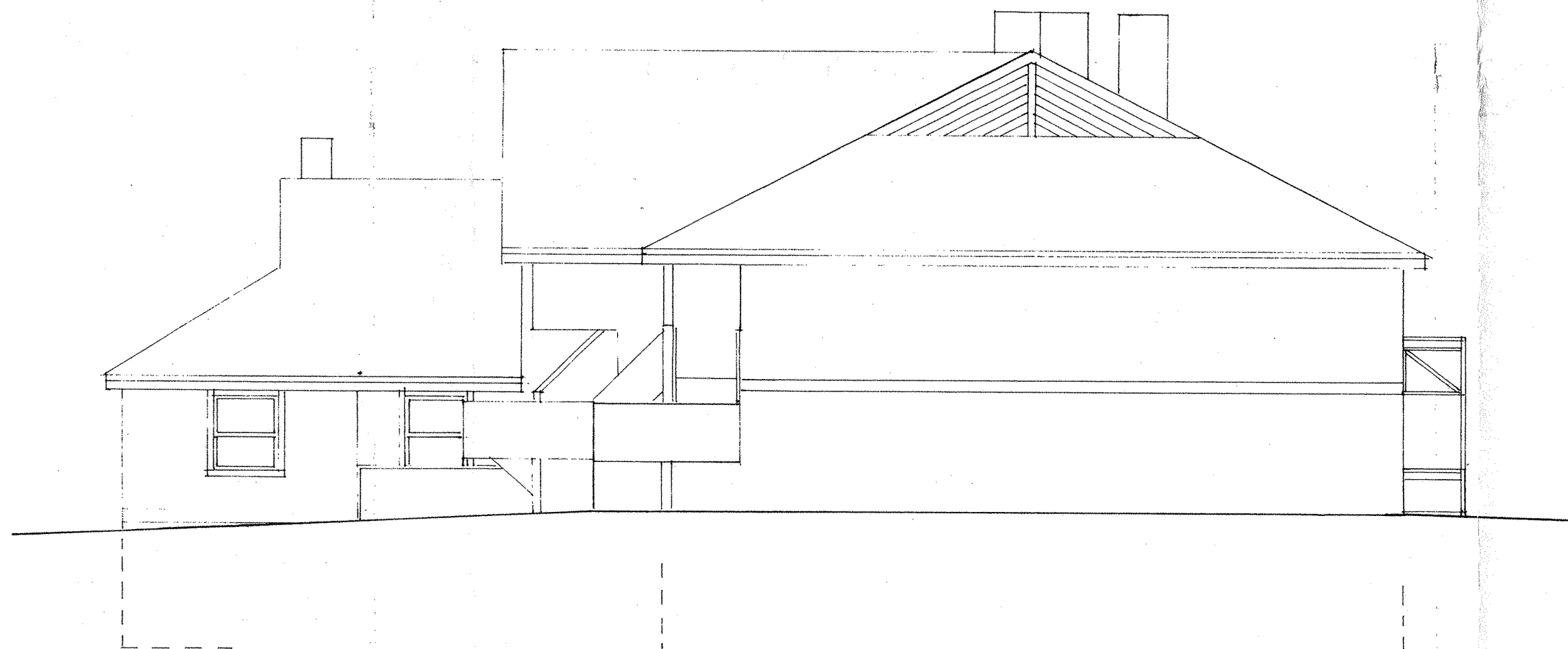
FASADE D - D
