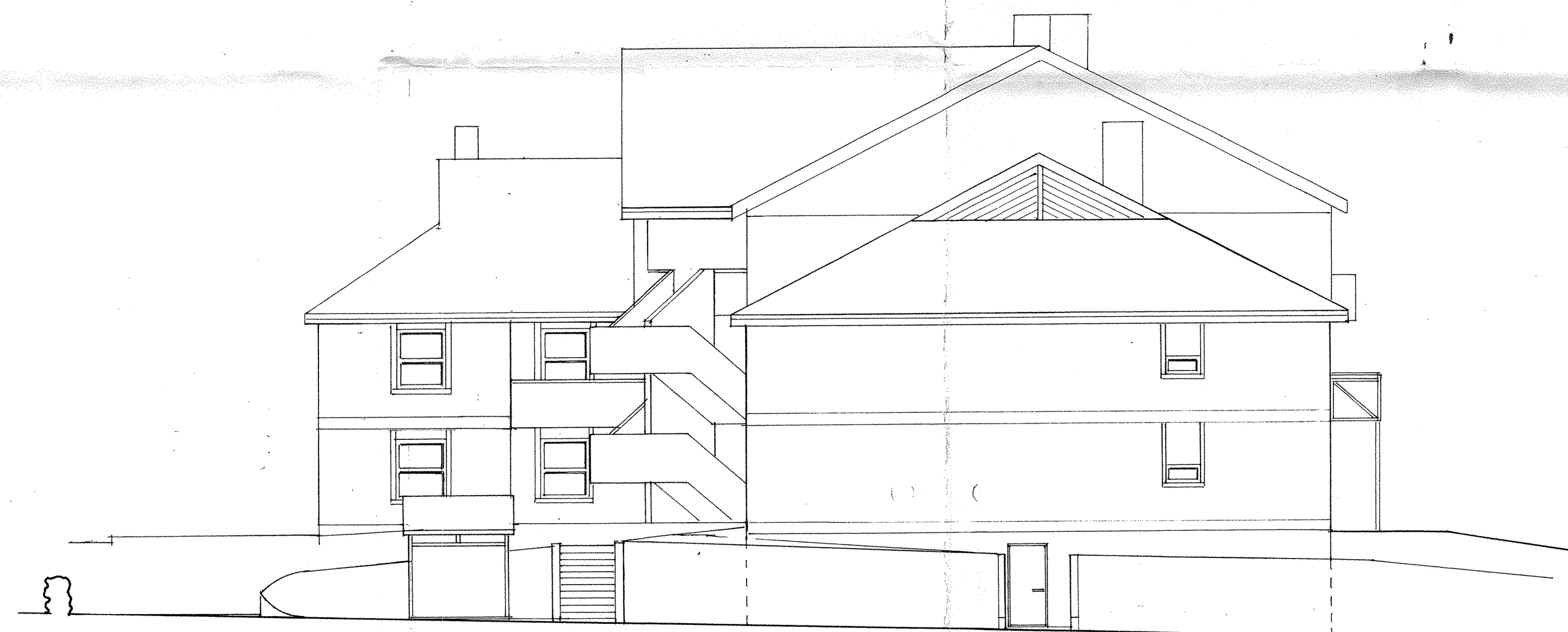
FASADE D - D
